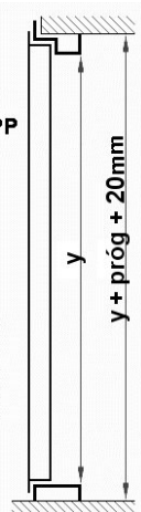
Podstawowe zależności wymiarowe Drzwi DC 3PP futryna ceowa
