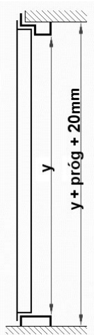
Podstawowe zależności wymiarowe Drzwi DC 3.1KT-M futryna kątowna
